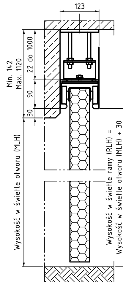
Montaż do sufitu podwieszony
