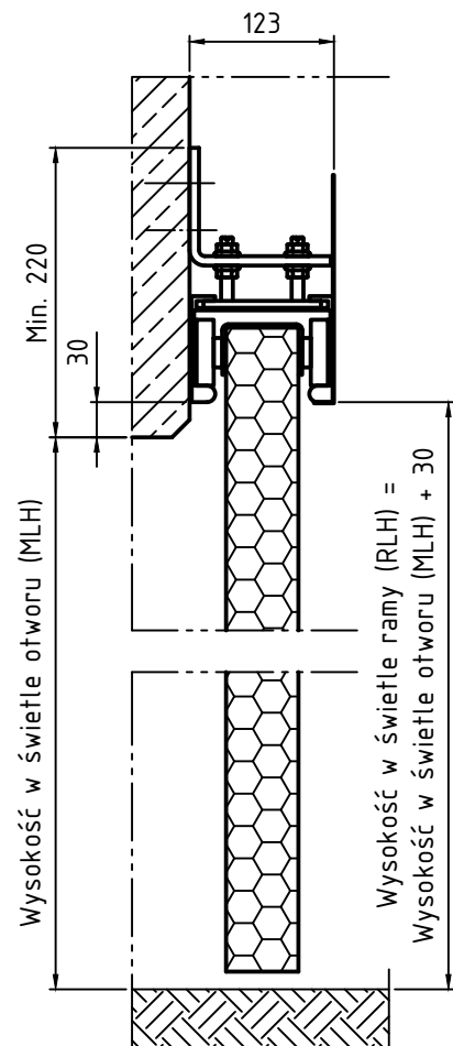
Montaż do ściany
