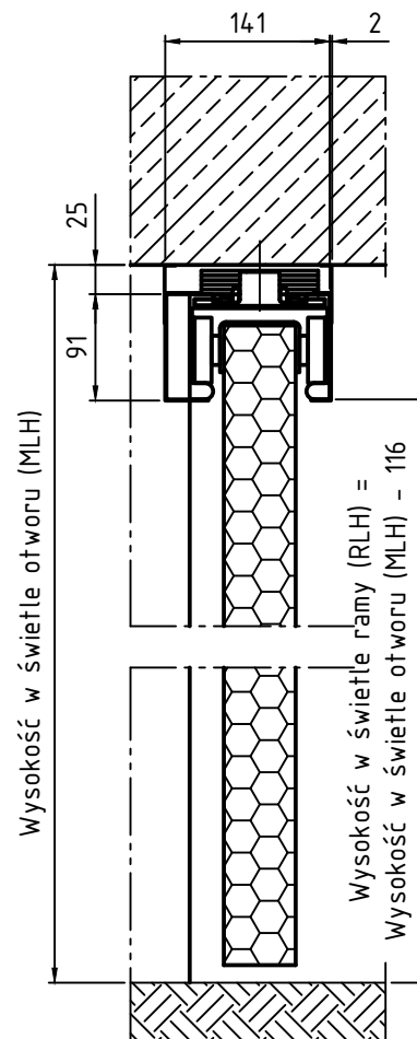
Montaż bezpośrednio do sufitu (z napędem)
