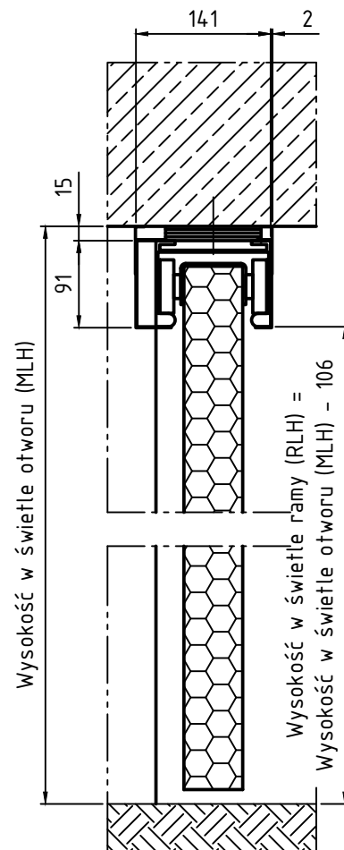
Montaż bezpośrednio do sufitu
