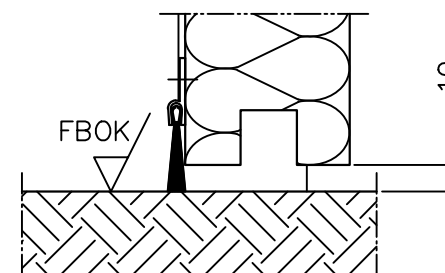
szczotka uszczelniająca
