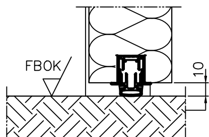
uszczelka opadająca
