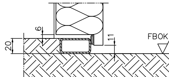
profil zamknięty 20 mm + skrzydło obwiedniowe, alternatywnie kątownik
