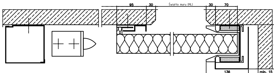
Brama przesuwna 1-skrzydłowa przeciwwaga po przeciwnej stronie (EI60) EI90 (EI120) ściana betonowa
