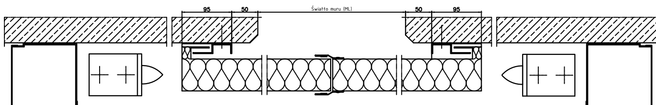
Brama przesuwna 2-skrzydłowa z przeciwwagą (EI60) EI90 (EI120) ściana betonowa
