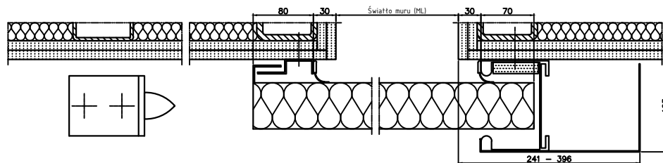
Brama przesuwna 1-skrzydłowa wlot normalny EI30 z dymoszczelnością ściana w systemie suchej zabudowy
