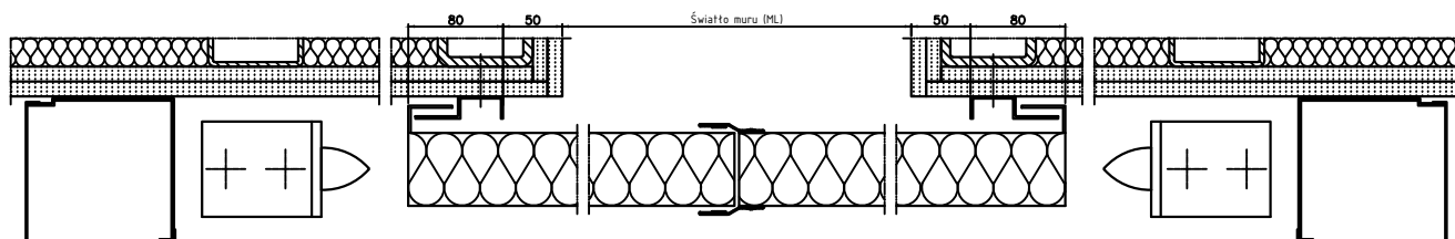
Brama przesuwna 2-skrzydłowa z przeciwwagą EI30 ściana w systemie suchej zabudowy
