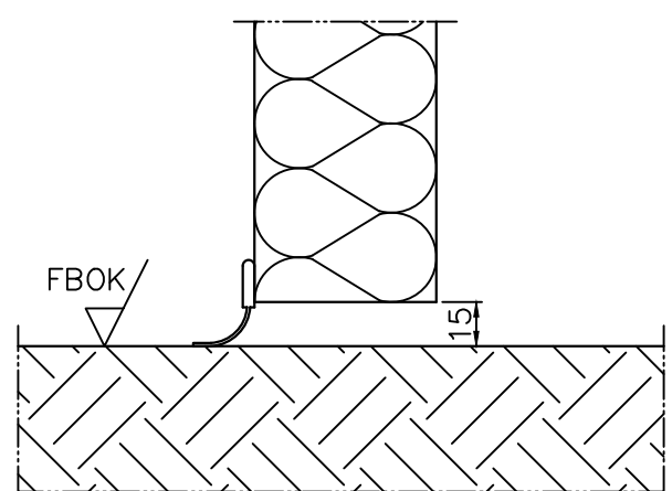
Detal progowy z dymoszczelnością
