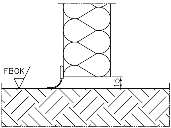
Detal progowy szczelina 15 mm
