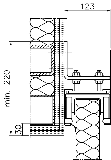
Montaż naścienny ściana w systemie suchej zabudowy z dymoszczelnością
