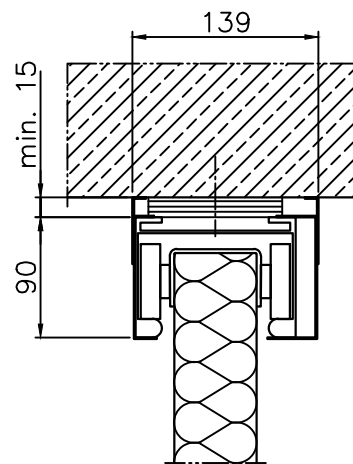
Montaż sufitowy bezpośredni ściana betonowa
