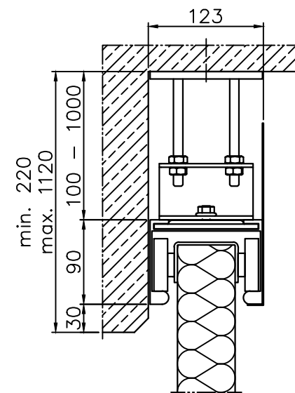
Montaż sufitowy podwieszany ściana betonowa
