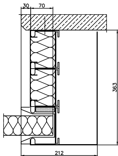
Włot normalny teleskop 3-częściowy ściana betonowa EI30
