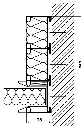
Włot w otworze teleskop 3-częściowy ściana betonowa EI30
